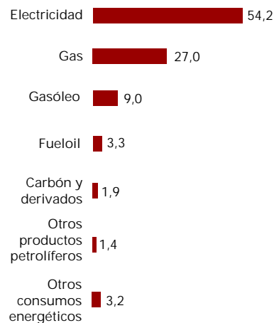
Consumos energéticos en la industria por tipo de consumo 2009 (%)
